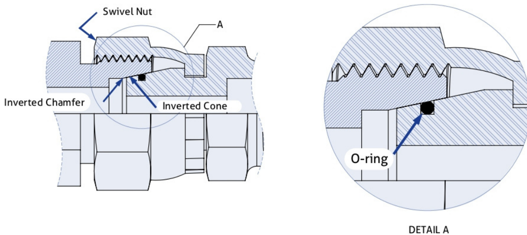
Figure 16: DIN Swivel Union
